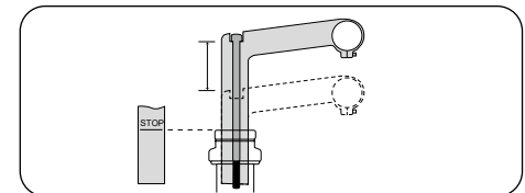
Höhenverstellung möglich
